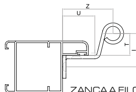
ZANCA A FILO (ZF)
