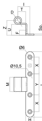
ZANCA A FILO (ZF)
