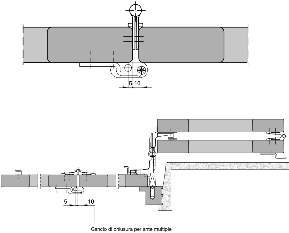
Gancio di chiusura per ante multiple
