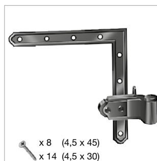
G550-30 Cerniera con squadretta 220x220 [set]
