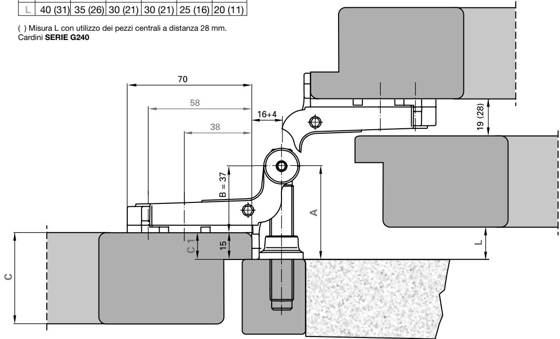
Cardini SERIE G240
