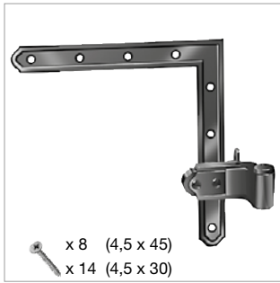
G560-30 Cerniera con squadretta 220x220 (set)
