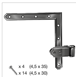
G440-30 Cerniera con squadretta 220x220 (set)
