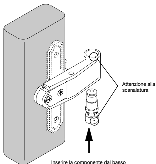
Inserire la componente dal basso
