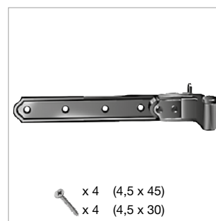
G560-40 Cerniera con bandella lunga
