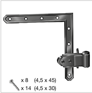
G540-30 Cerniera con squadretta 220x220 (set)
