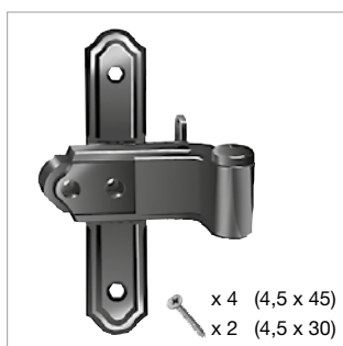
G460-20 Cerniera con bandella a croce
