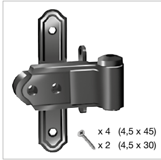
G540-20 Cerniera con bandella a croce
