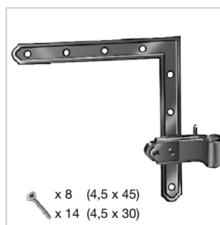
G460-30 Cerniera con squadretta 220x220 [set]
