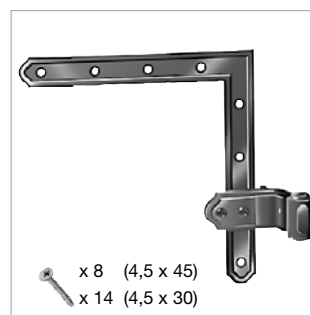
G300-3... Cerniera con squadretta 220x220 (set)
