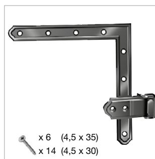
G400-30 Cerniera con squadretta 220x220 [set]
