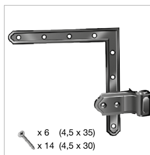
G420-30 Cerniera con squadretta 220x220 [set]
