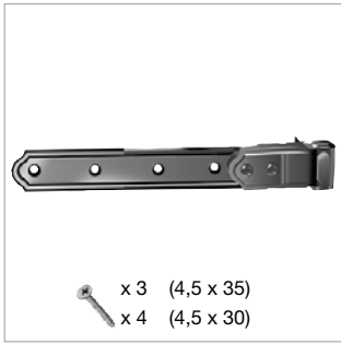
G410-40 Cerniera con bandella lunga
