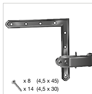
G570-30 Cerniera con squadretta 220x220 [set]
