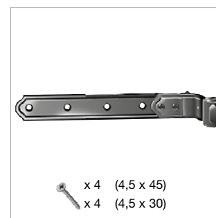
G300-4... Cerniera con bandella lunga
