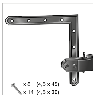
G530-30 Cerniera con squadretta 220x220 [set]
