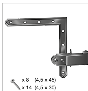
G500-30 Cerniera con squadretta 220x220 [set]
