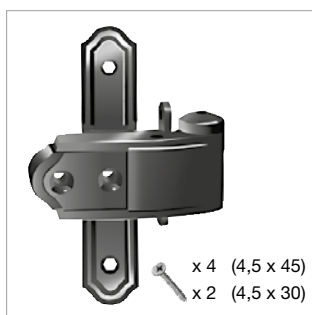
G530-20 Cerniera con bandella a croce
