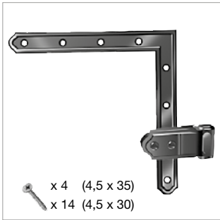
G430-30 Cerniera con squadretta 220x220 (set)
