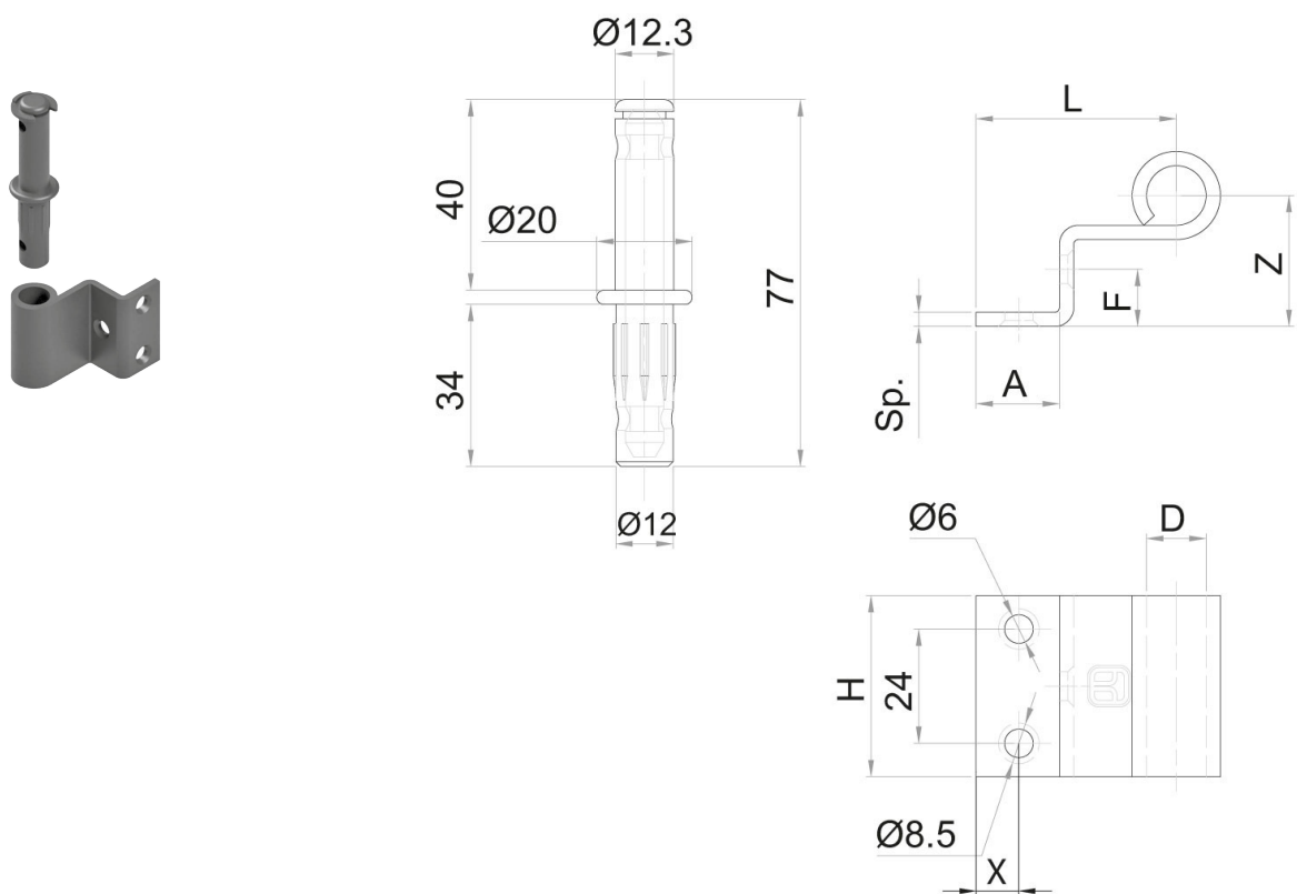
SERIE 471 Bandella diritta occhio laterale esterno doppia zanca con perno H=38
