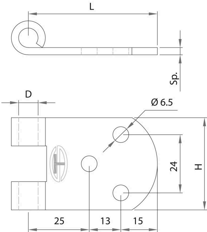
SERIE 445 Bandella alla "vicentina" H=38
